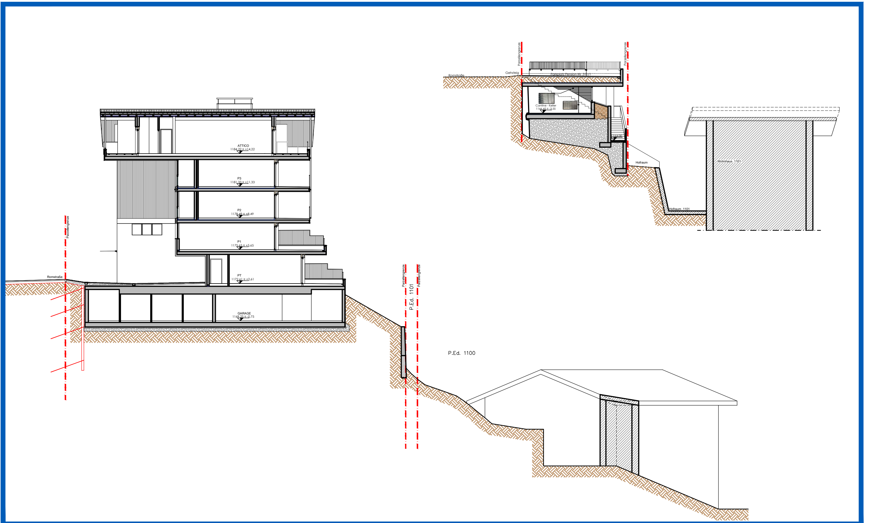
Sezione trasversale e Sezione cantine - Querschnitt und Sektion keller 1:200
