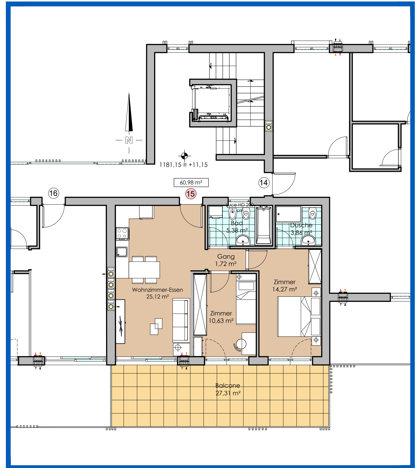
3 Stock - Piano Terzo 1:100 Wohnung 15 Appartamento
