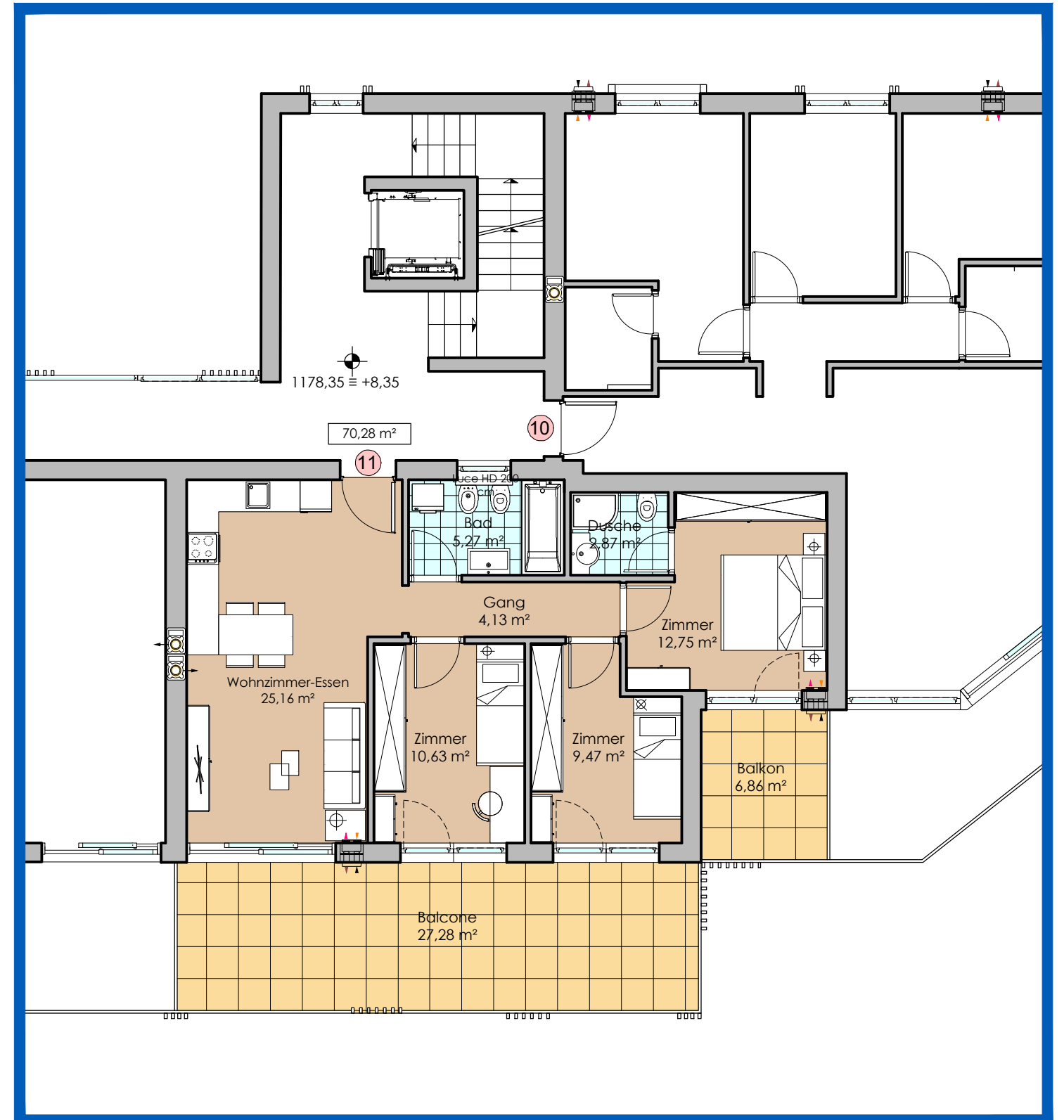
2 Stock - Piano Secondo 1:100 Wohnung 11 Appartamento
