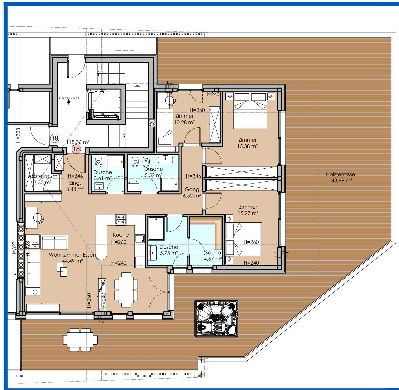
Dachgeschoss - P. Attico 1:100 Wohnung 18 Appartamento
