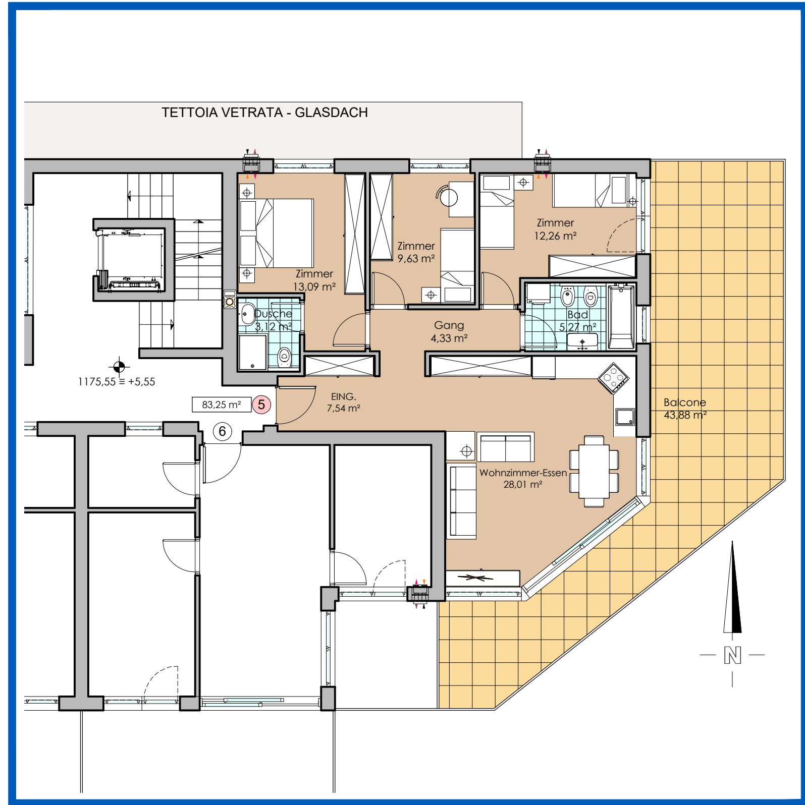
1 Stock - Piano Primo 1:100 Wohnung 5 Appartamento
