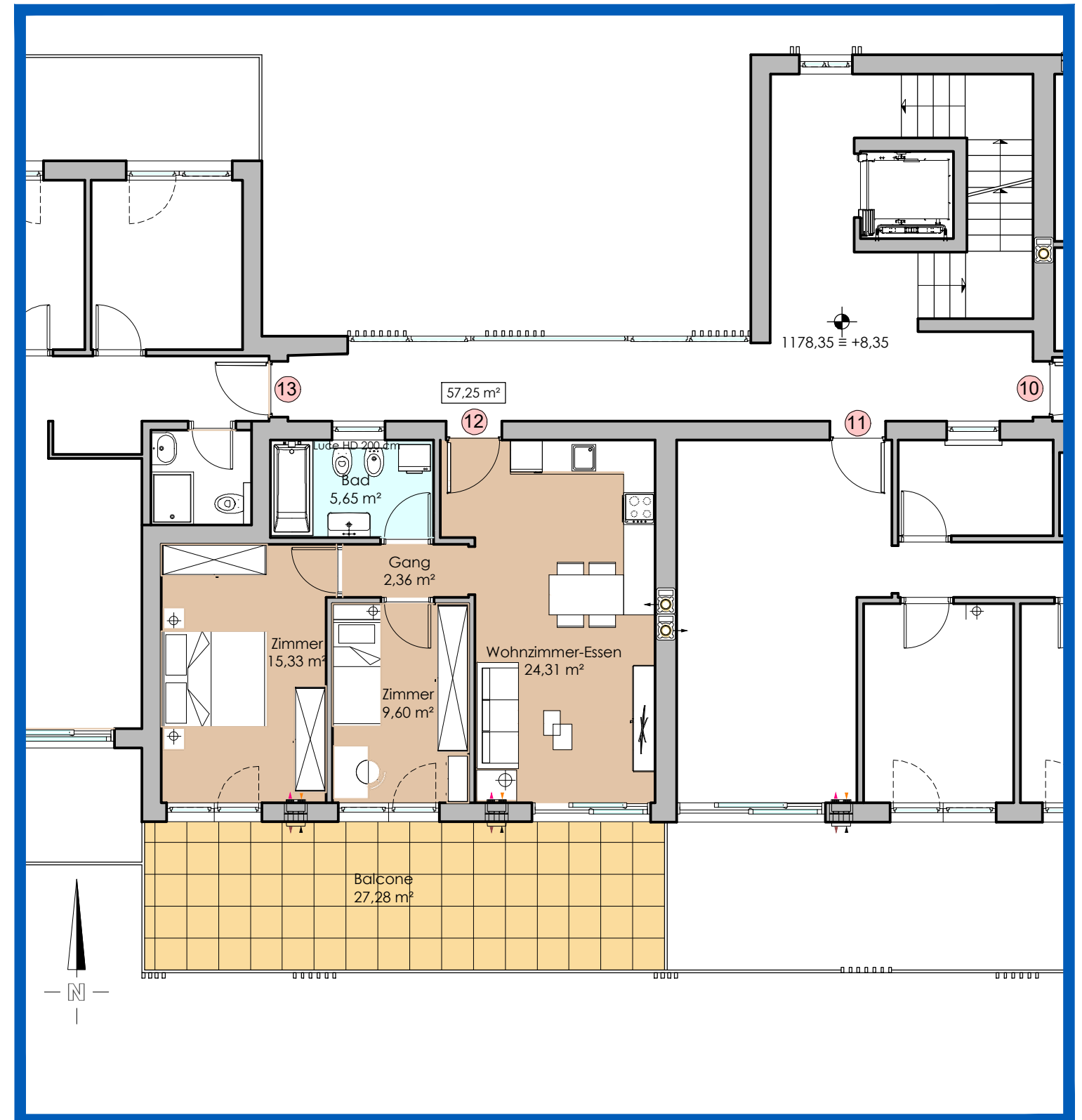
2 Stock - Piano Secondo 1:100 Wohnung 12 Appartamento
