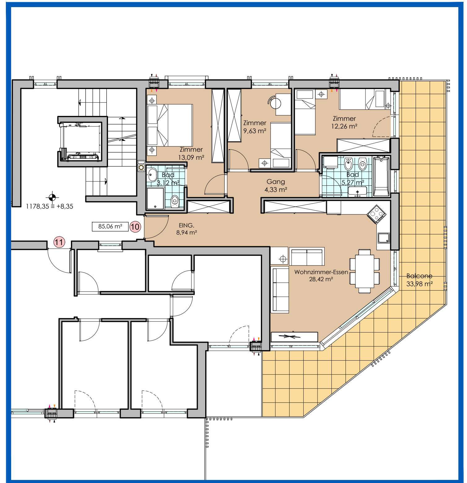
2 Stock - Piano Secondo 1:100 Wohnung 10 Appartamento
