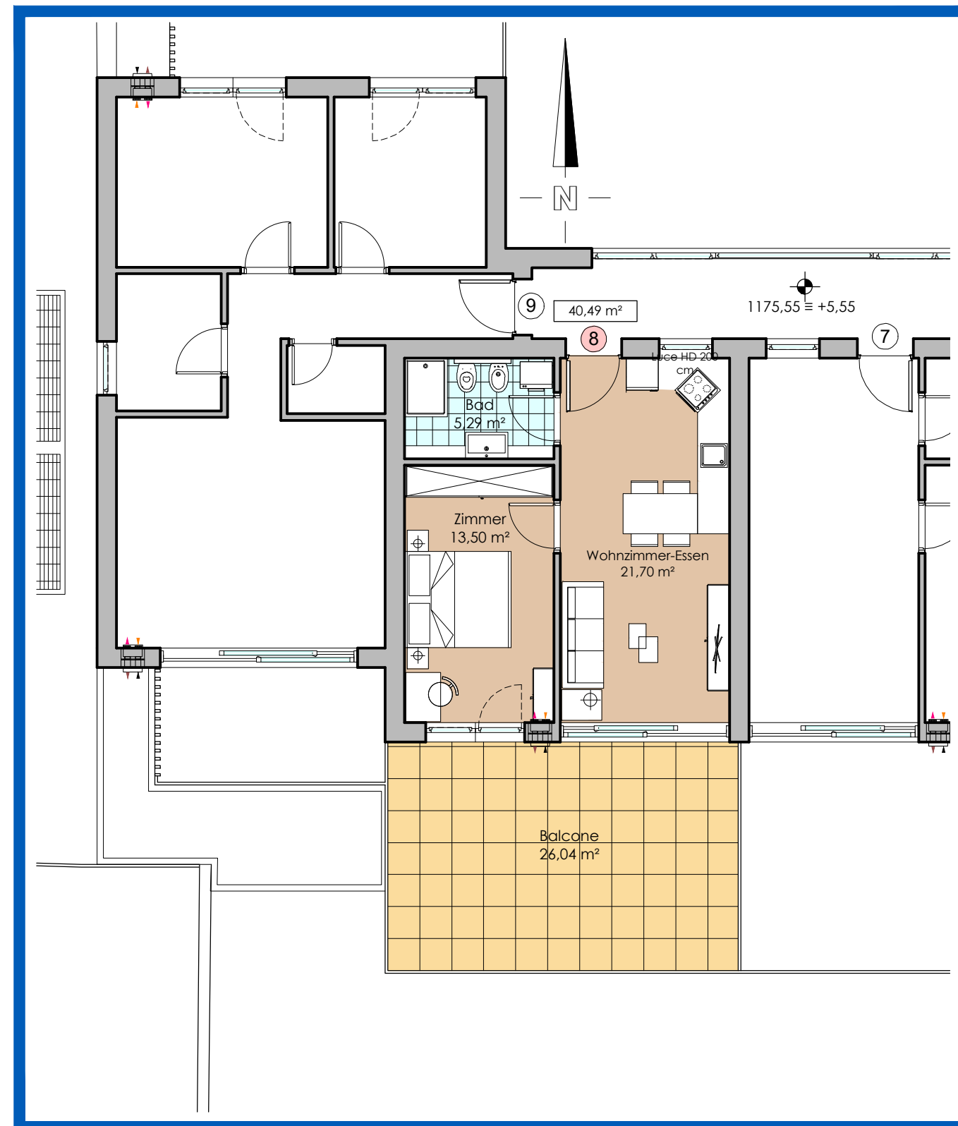
1 Stock - Piano Primo 1:100 Wohnung 8 Appartamento
