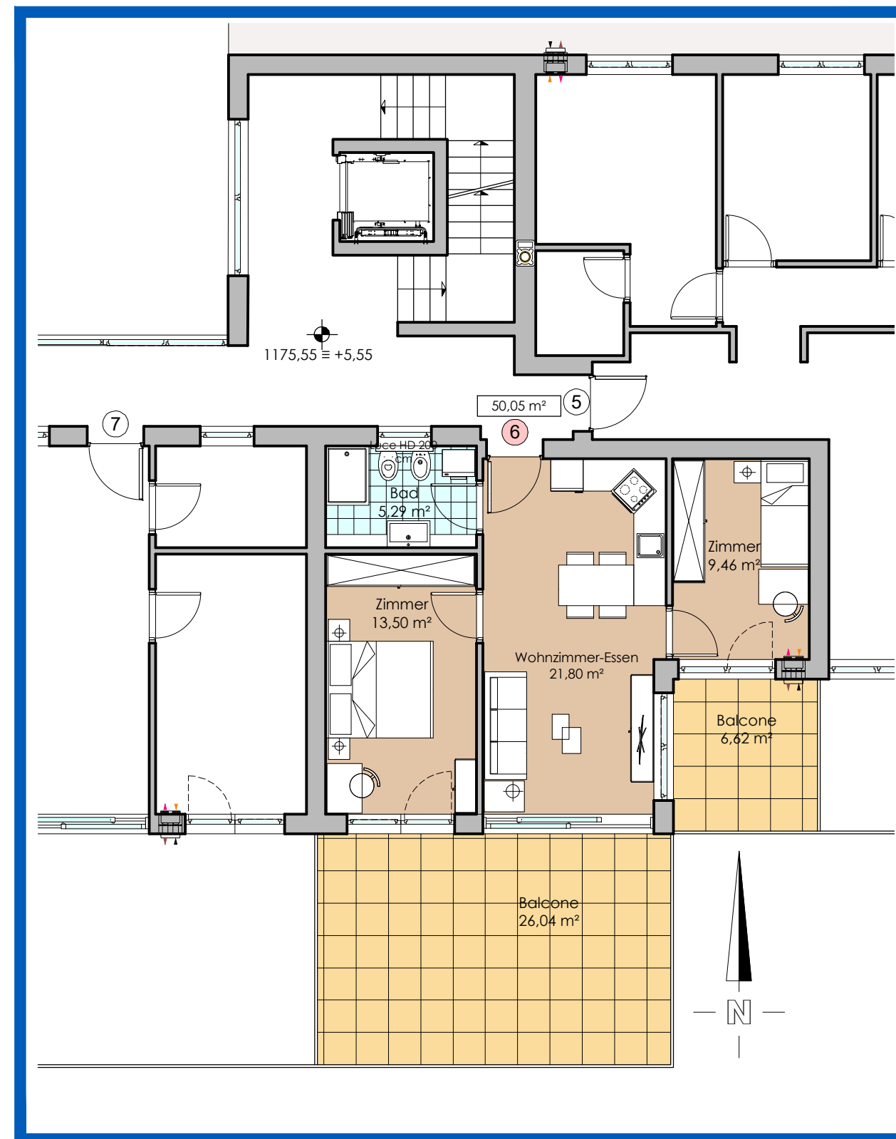
1 Stock - Piano Primo 1:100 Wohnung 6 Appartamento
