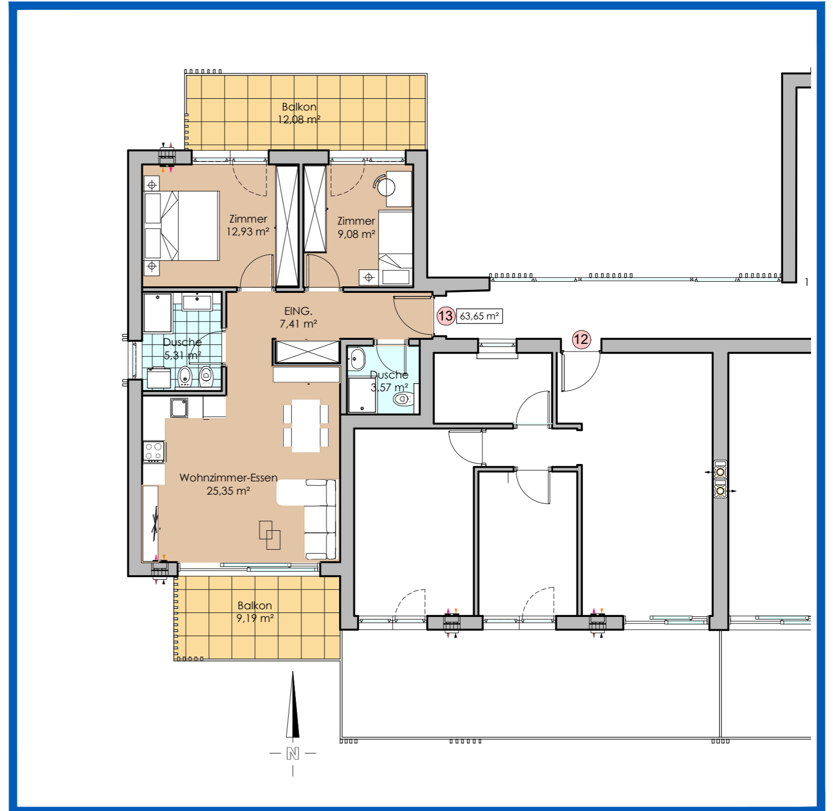
2 Stock - Piano Secondo 1:100 Wohnung 13 Appartamento
