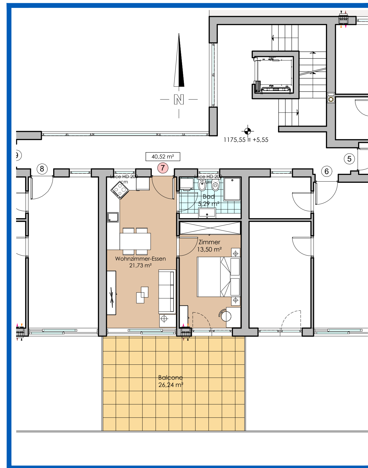
1 Stock - Piano Primo 1:100 Wohnung 7 Appartamento
