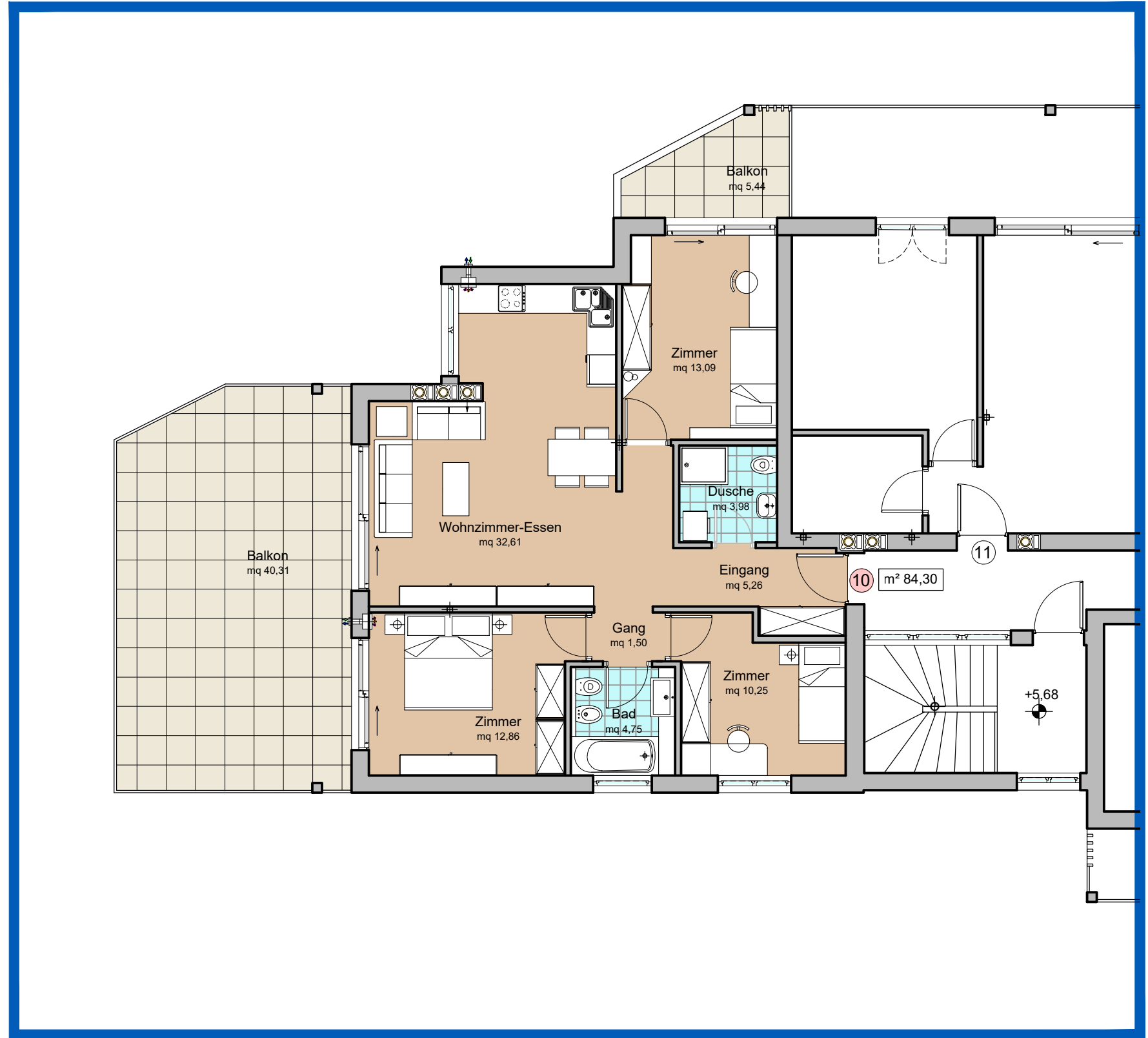
2.Obergeschoss - Secondo Piano Wohnung - Appartamento 10 - 1:100
