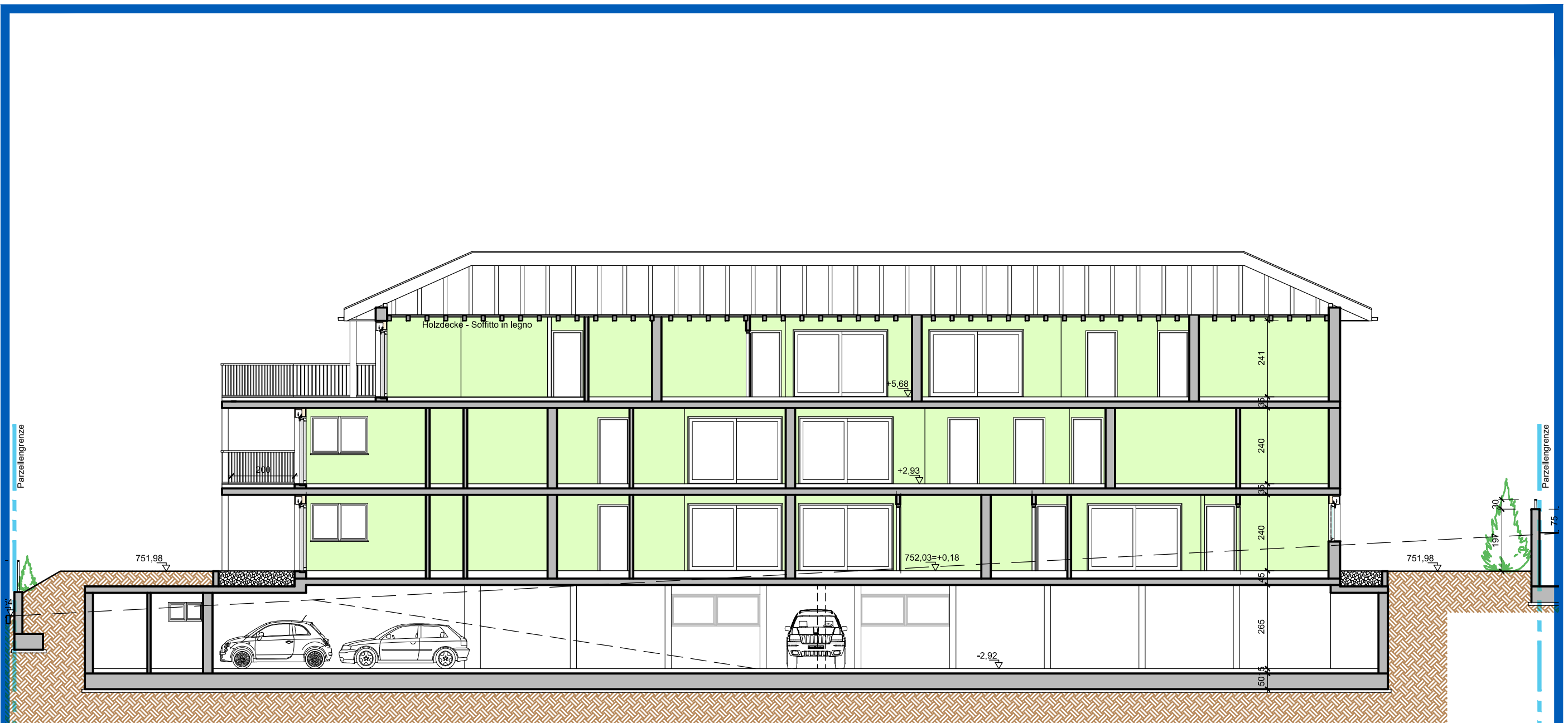
SCHNITT A-A
