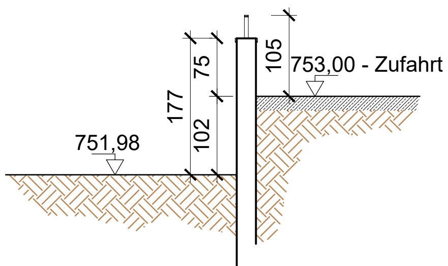
Sez. 6 Schnitt
