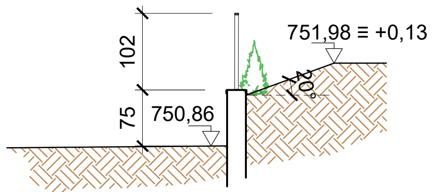
Sez. 3 Schnitt
