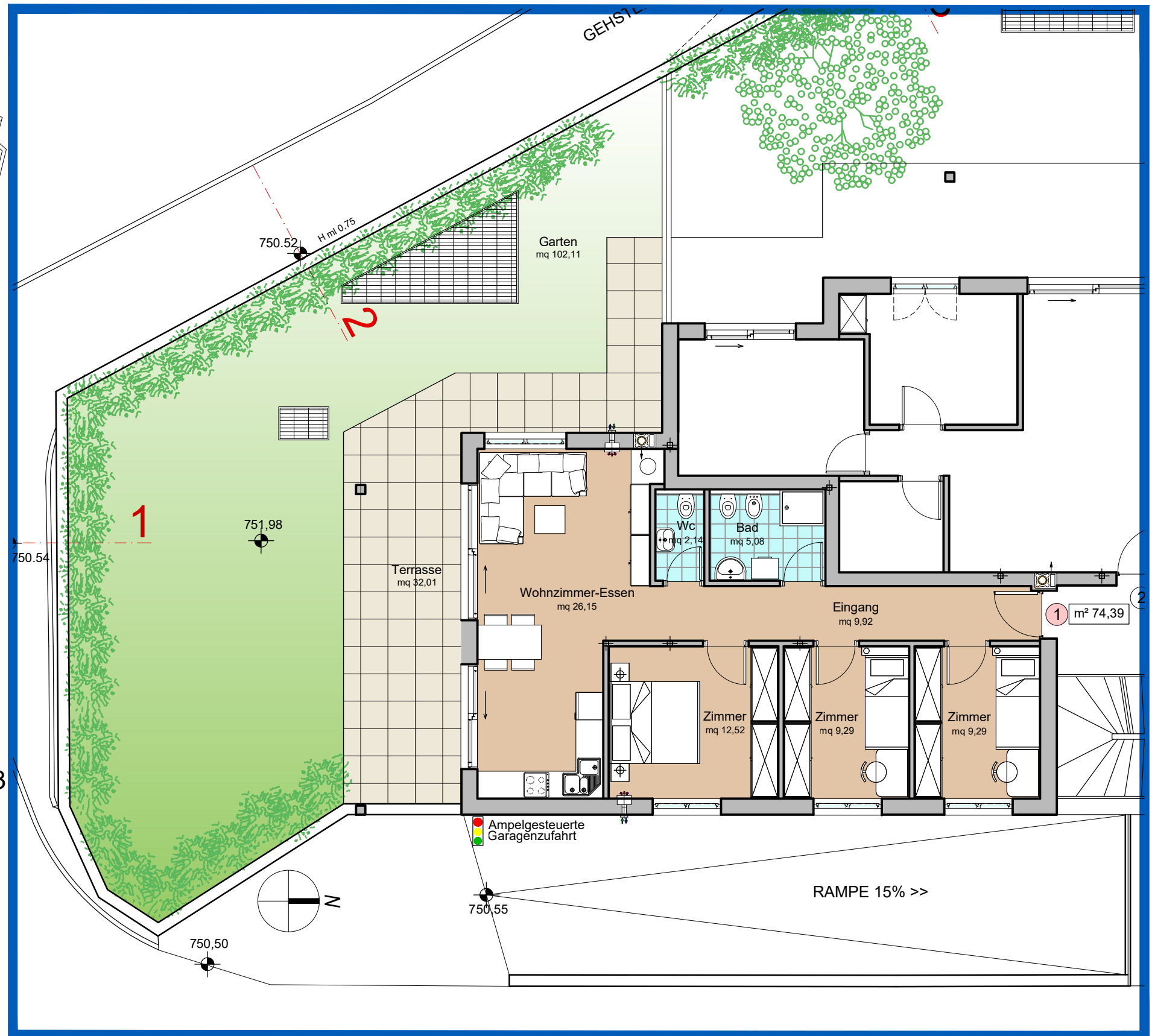
Erdgeschoss - Piano Terra Wohnung - Appartamento 1- 1:100
