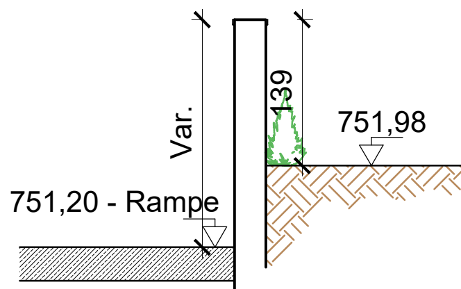
Sez. 5b Schnitt
