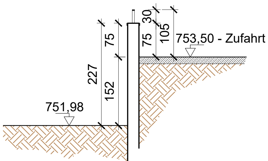
Sez. 7 Schnitt
