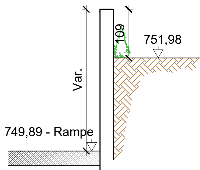
Sez. 5a Schnitt
