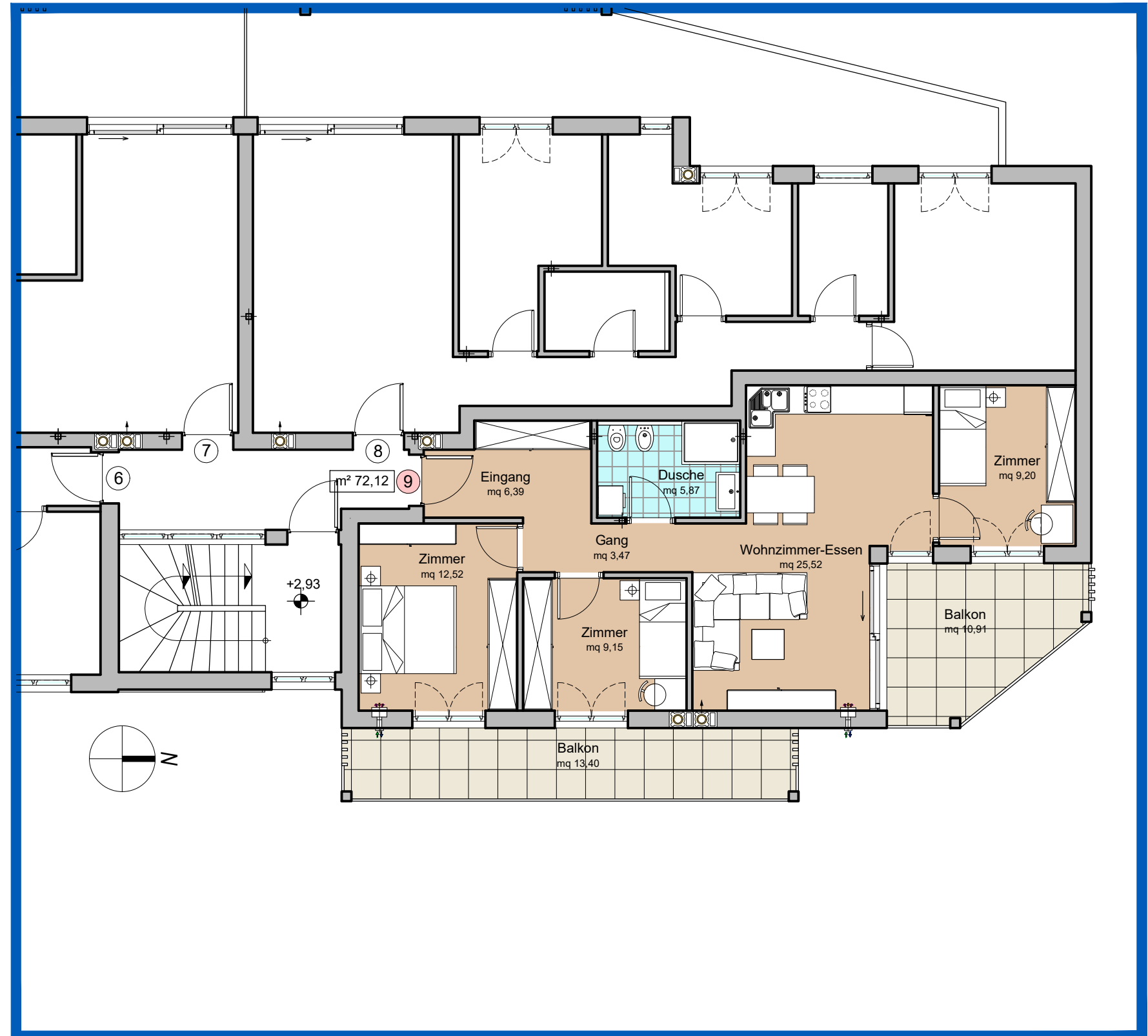
1. Obergeschoss - Primo Piano Wohnung - Appartamento 9 - 1:100
