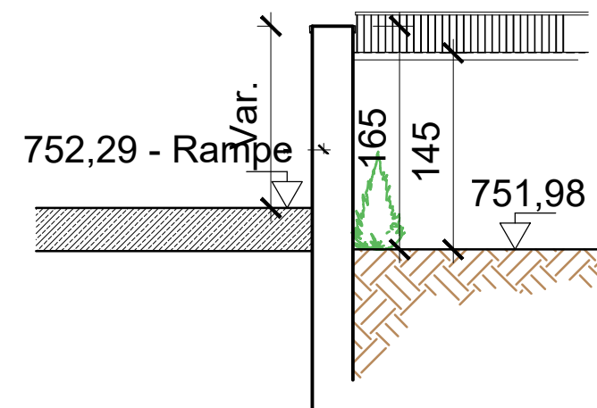
Sez. 5c Schnitt
