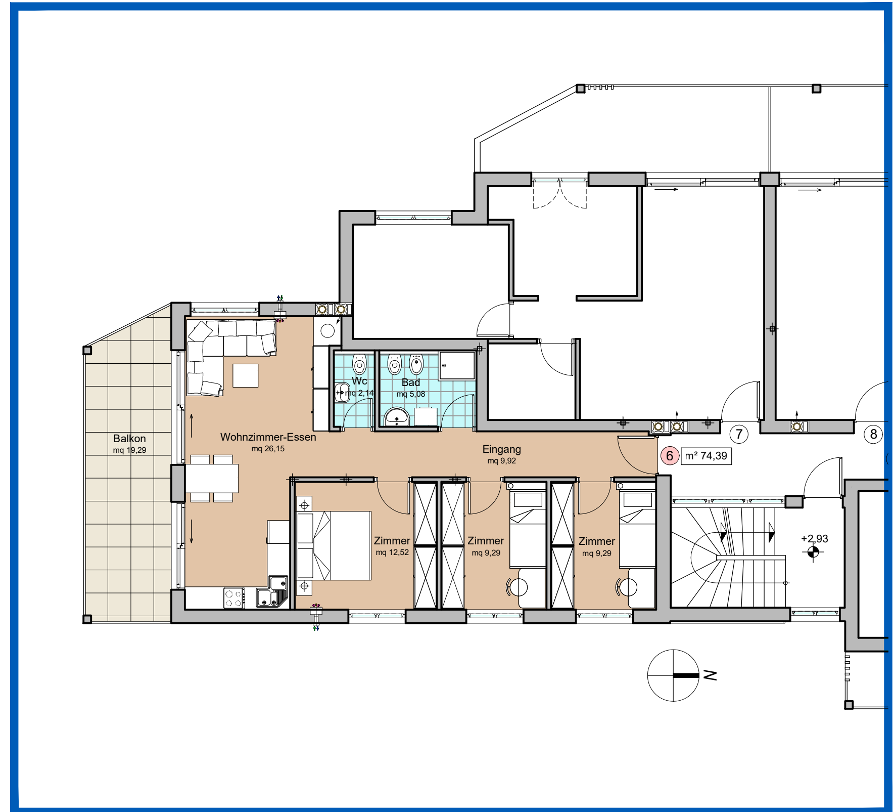
1. Obergeschoss - Primo Piano Wohnung - Appartamento 6 - 1:100
