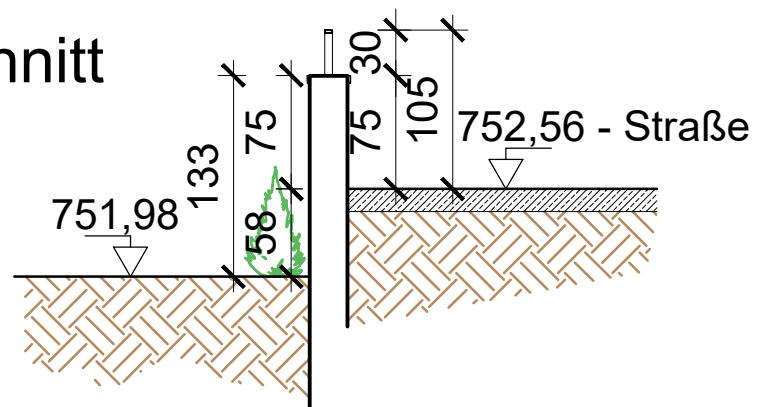
Sez. 8 Schnitt
