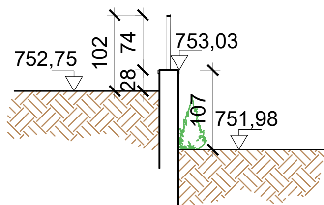
Sez. 4 Schnitt
